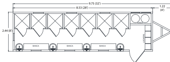
REGADERAS MM832
